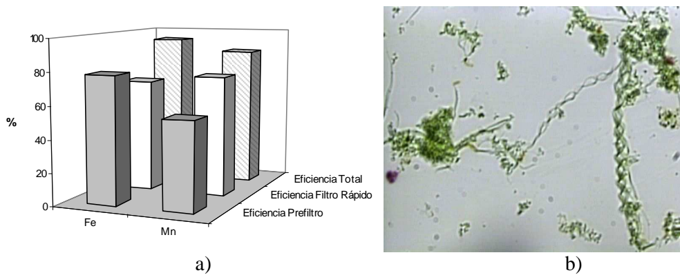
Figura 10 – Eficiencias remoción de Fe y Mn, b) Microfotografía (1000x) de bacterias del Fe en barro de lavado Planta Florencia.
